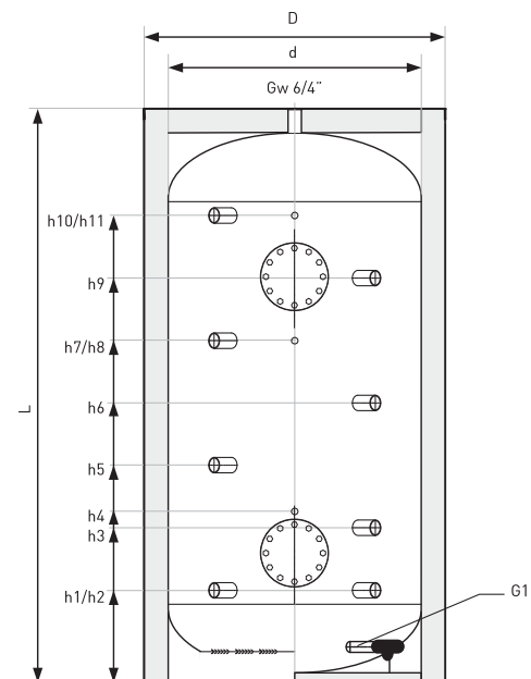
Schéma zásobníků 3000 - 5000l
