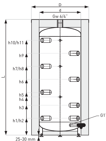
Schéma zásobníků 300 - 2000l
