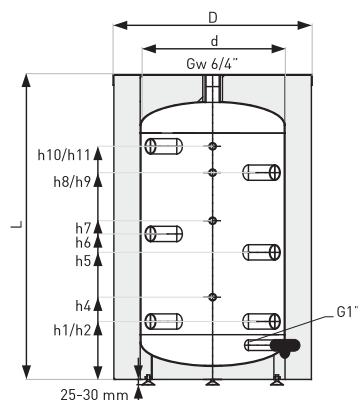
Schéma zásobníku 200l
